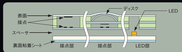
構造図
