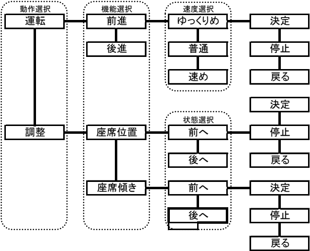
<車イス制御>
