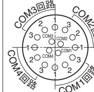
端子番号図
