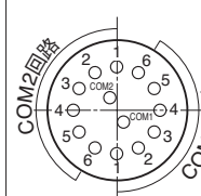
端子番号図
