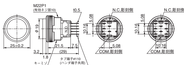
全面照光形 (白熱球・LED)
