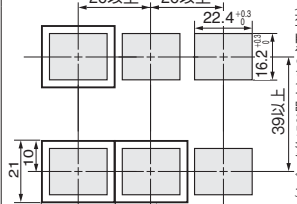
取付穴寸法図
