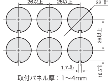
連続取付け
