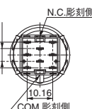
2極双投
