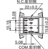
単極双投
