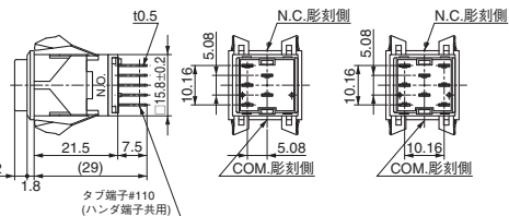
単極双投
