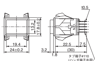
端 子 部
