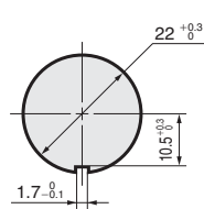
単体取付け
