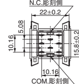
2極双投
